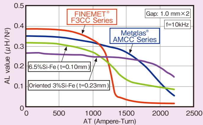
図1 各種カットコアの直流重量特性* Fig. 1 DC superposition characteristics of various cut cores*
